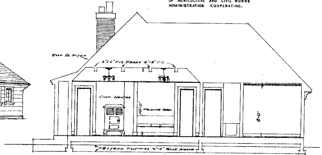
• LONGITUDINAL SECTION •
